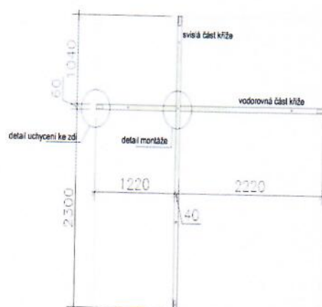
POHLED M 1:50
