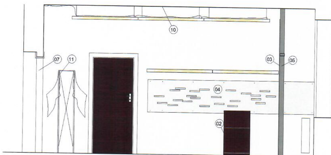
POHLED B M 1:50
